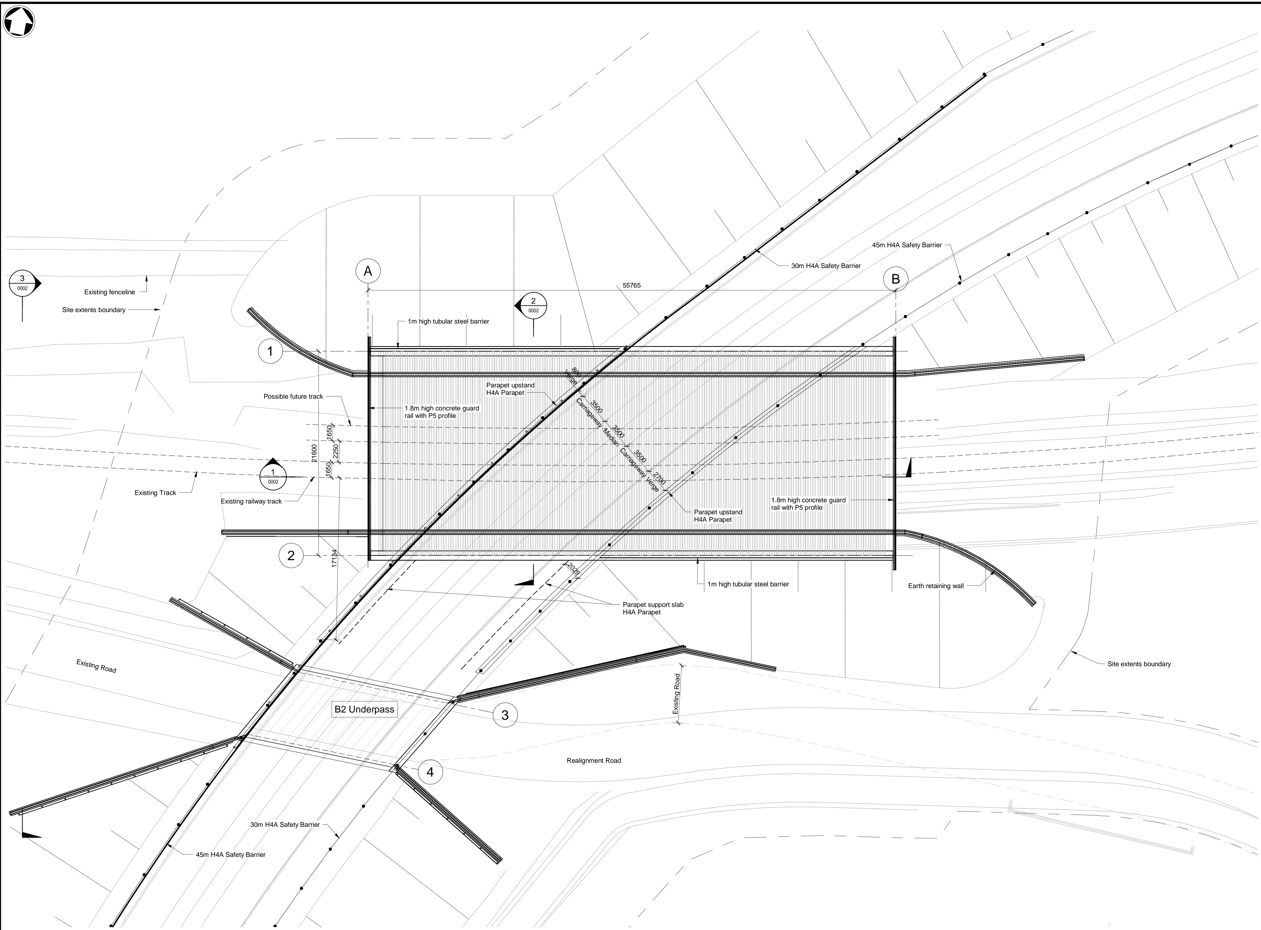
Plan 1 : 200
