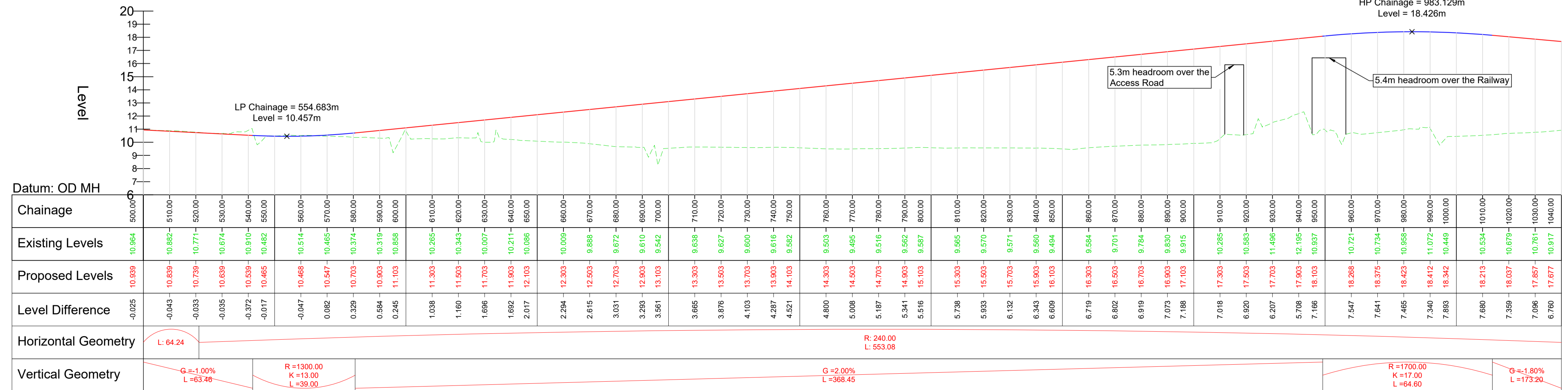
M-ML-RE-XX-03_2 SCALE: H 1:1000,V 1:200. DATUM: 6.000
